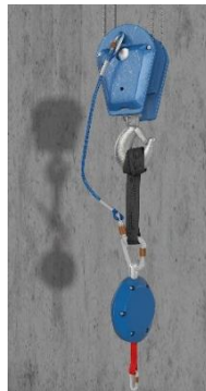
Bild 3: Redundante Sicherung
